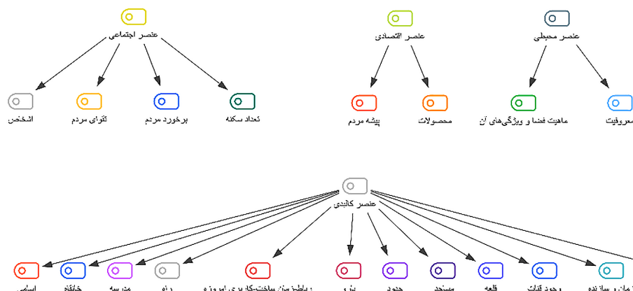
تصویر ۱. نمودار درختی حاصل از دسته‌بندی عناصر.
